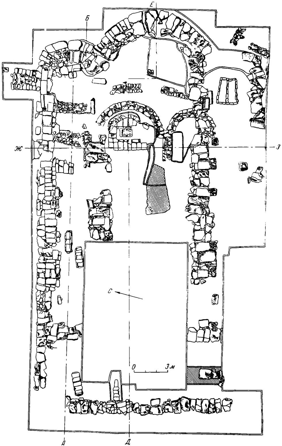
Рис. 6. Поселение у с. Планерское. План базилики (по В. П. Бабенчикову).
