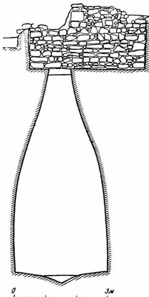
Рис. 8. Цистерна бутылковидной формы для хранения вина. Участок И.
