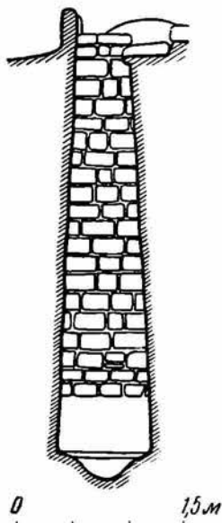
Рис. 14. Разрез каменного водосборного колодца дома № 3 эллинистического времени. Участок АГД.
